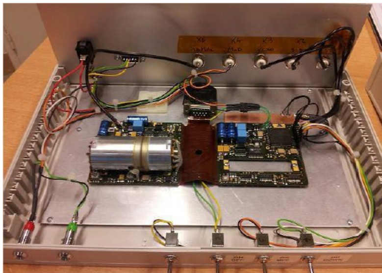
Vue de l'horloge à Rb pédagogique
